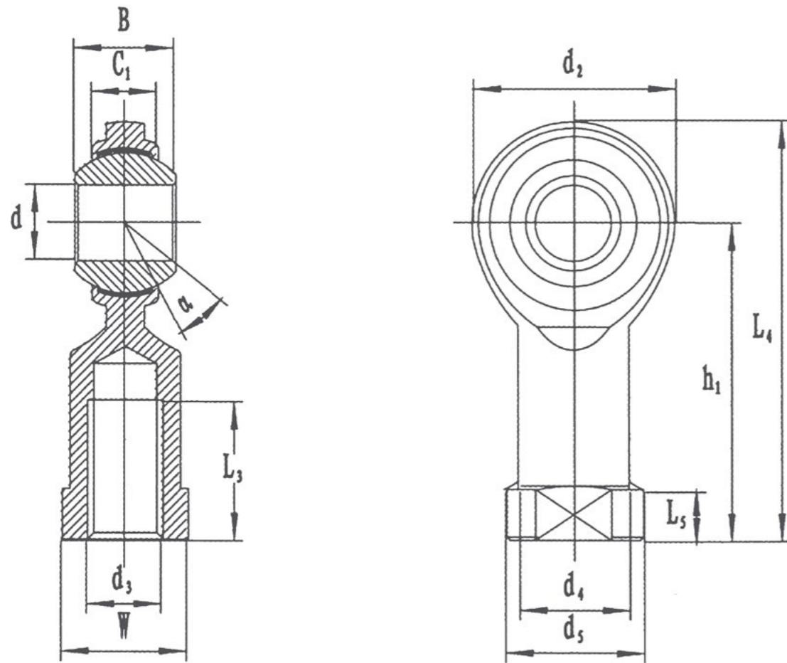
Gelenkkopf NHS mit Innengewinde.
