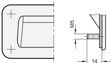
Montageausbruch
