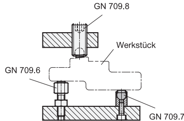
Anwendungsbeispiel verschiedener Pendelelemente mit O-Ring
