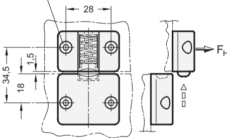
Montagehinweis / Bohrbild
