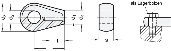
Bundschraube GN 732.1 als Lagerbolzen
