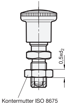
Raststift eingezogen
