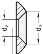
Bohrung für Senkschraube DIN 7991 / DIN ISO 2009
